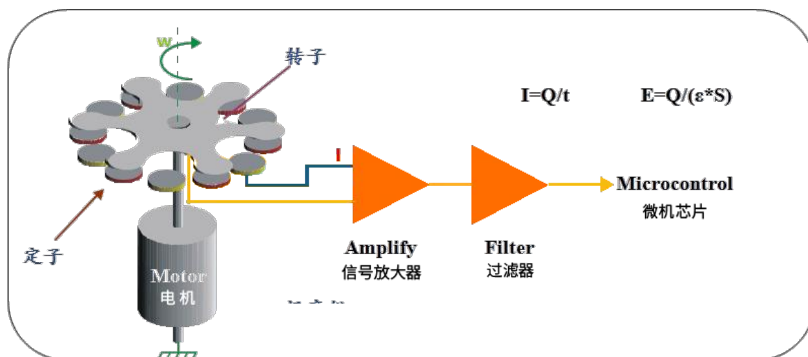
场磨式大气电场仪测量原理模型
